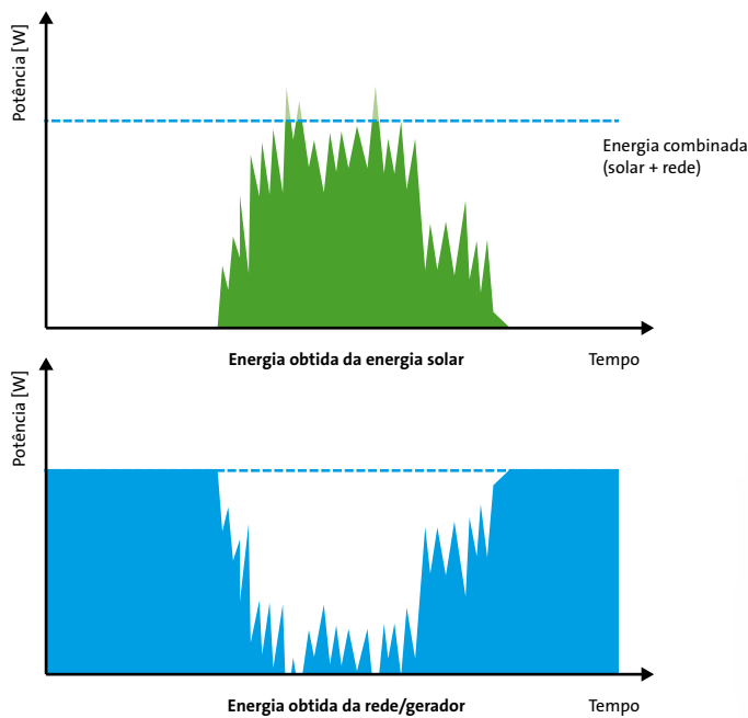
Figura 1: Operação de combinação de energia (dados fictícios).
