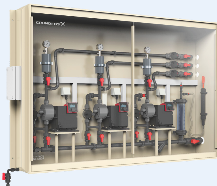
Exemple d'armoire FIT
