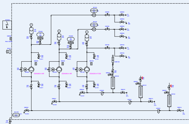
Exemple PID d'armoire sur mesure
