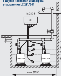
Стационарная установка с двумя насосами и шкафом управления LC 231/241
